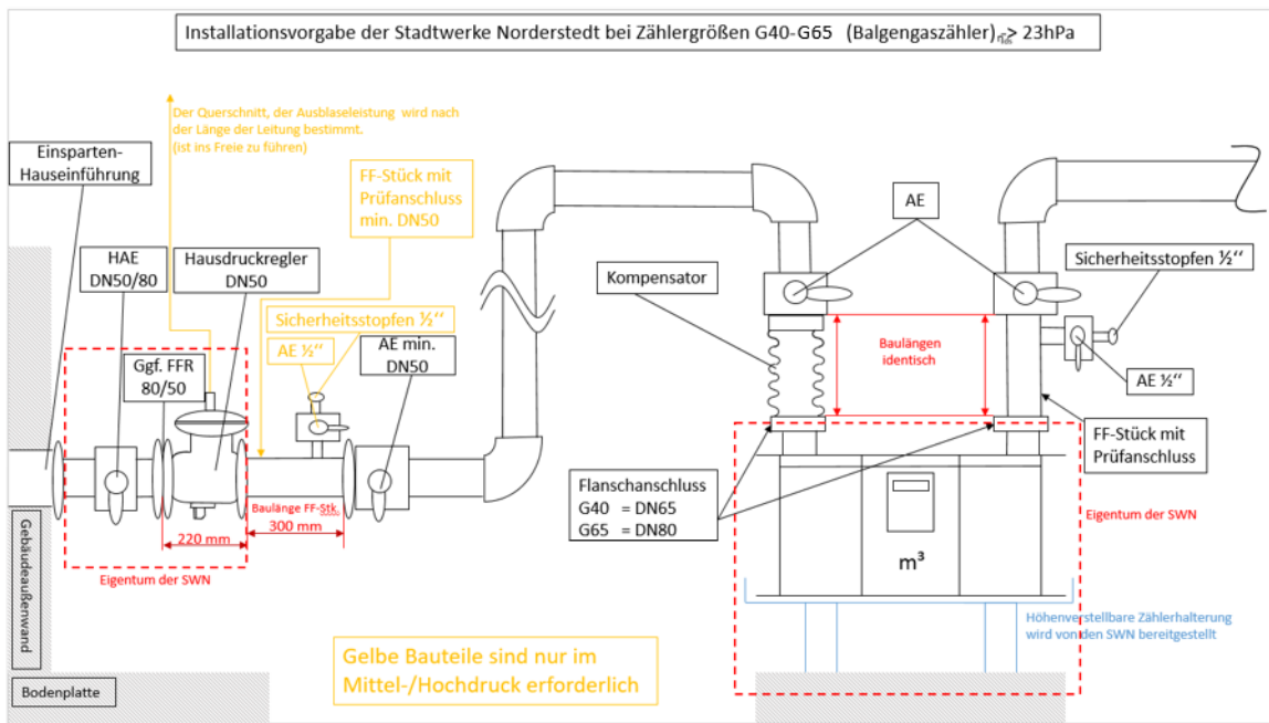
Abbildung 3 : Übersicht Gasmessung G40-G65
