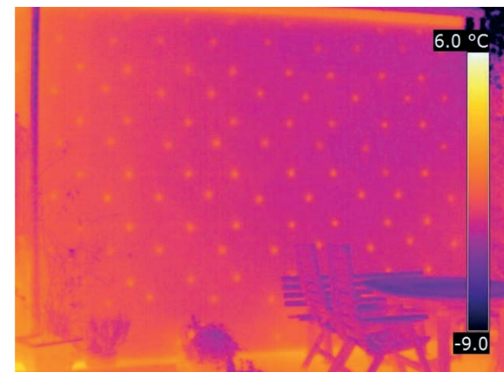
Dalmatiner-Effekt durch die Dübel beim Wärmedämmverbundsystem (WDVS)
