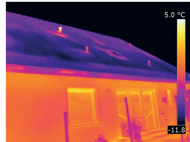
Luftundichtigkeit beim Dach
