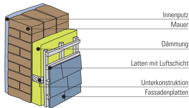
Außenwand mit Vorhangfassade
