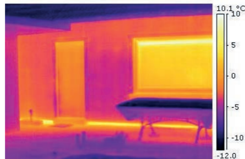
Thermografie eines nicht gedämmten Sockelanschlusses
