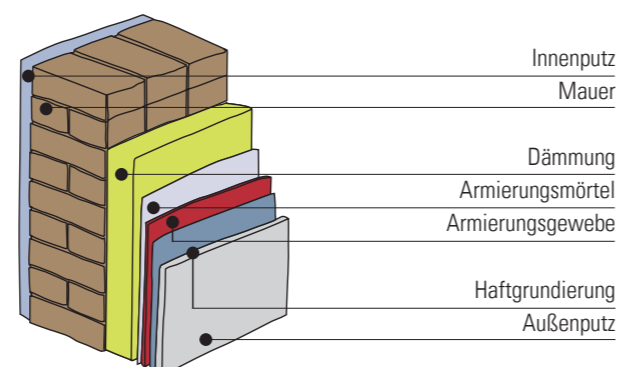
Außenwand mit Wärmedämm-Verbundsystem (WDVS)
