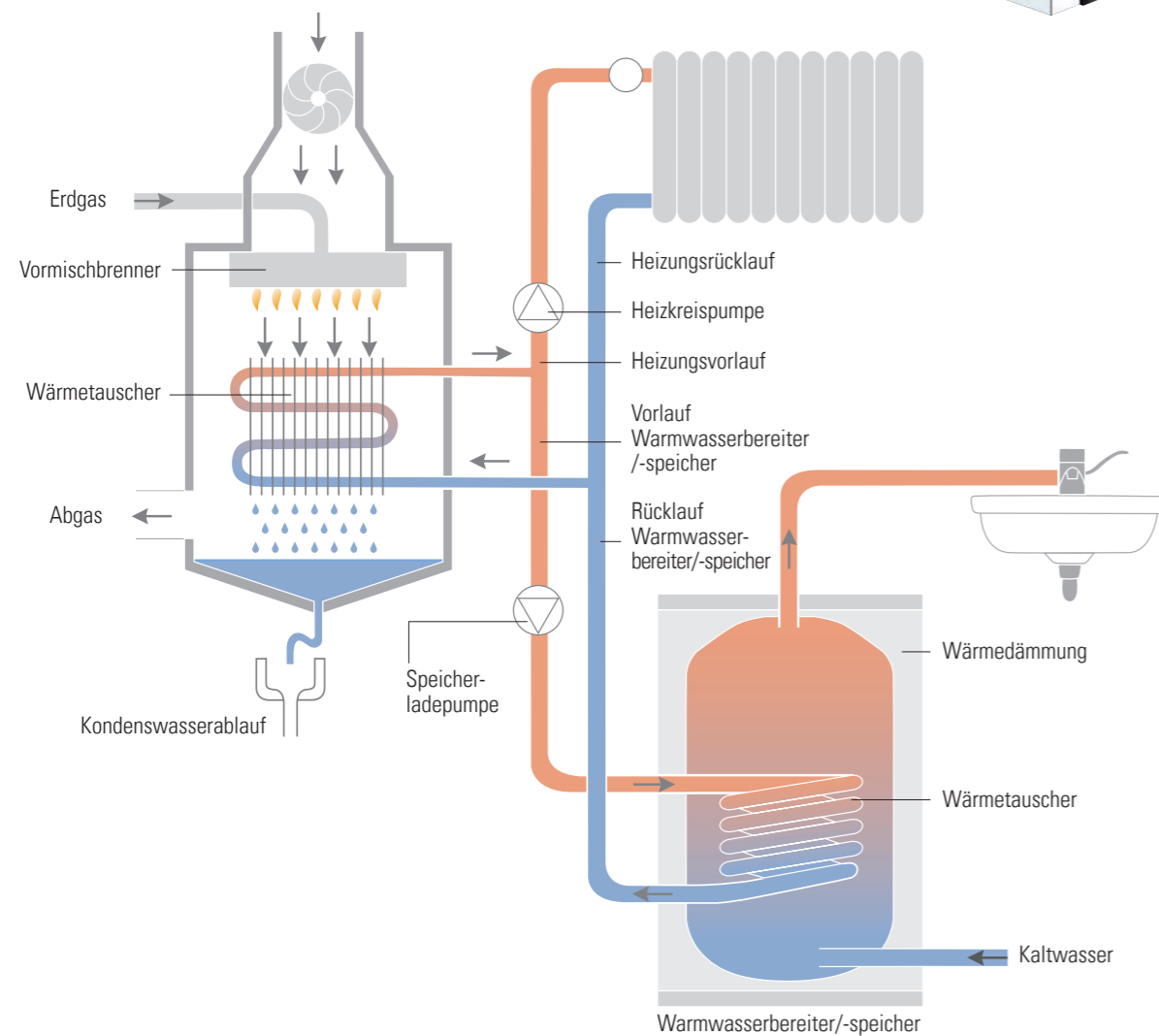
Heizung mit Brennwertkessel und Warmwasserbereitung
